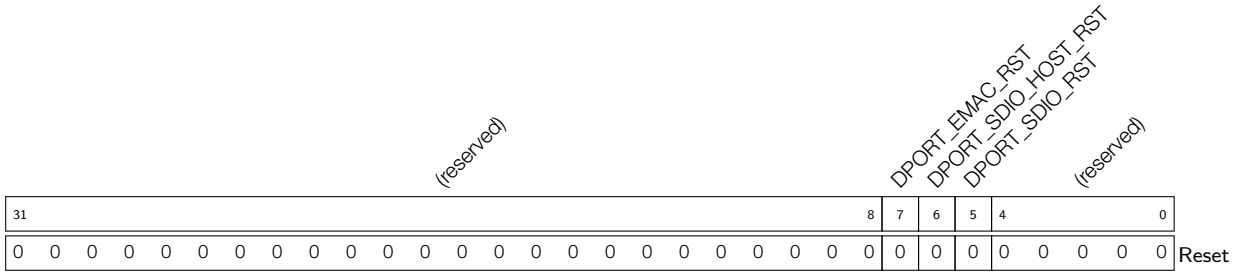
Register 5.20: DPORT_WIFI_RST_EN_REG (0x0D0)
