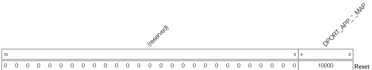
DPORT_APP*_MAP Interrupt map. (R/W)
