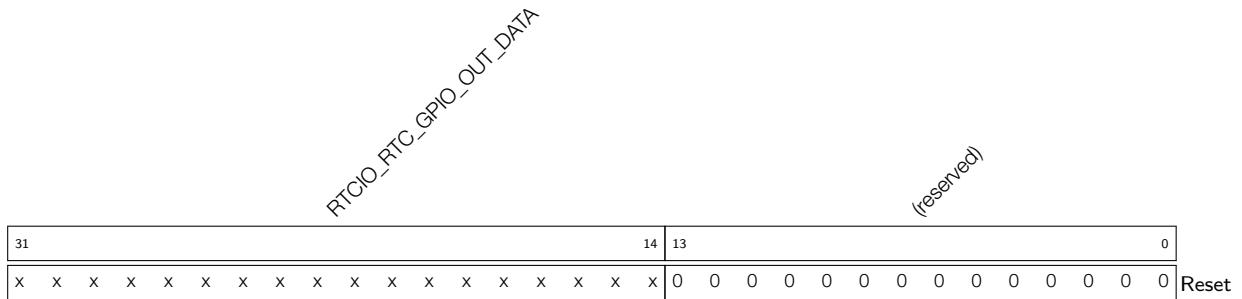
Register 4.35: RTCIO_RTC_GPIO_OUT_REG (0x0000)
