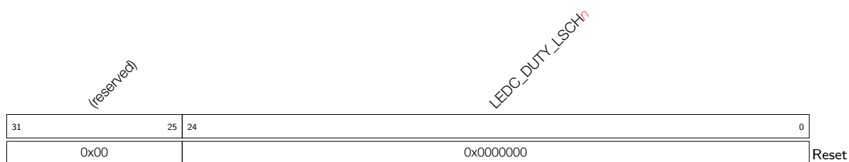
Register 14.8: LEDC_LSCH n _DUTY_REG ( n : 0-7) (0xC4+0x10* n )
